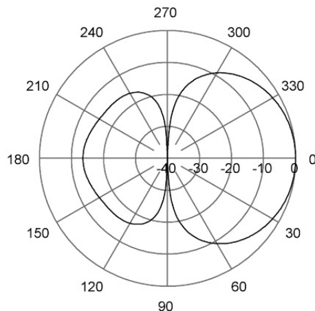
E-Plane | 445 MHz
