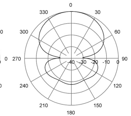
H-Plane | 160 MHz
