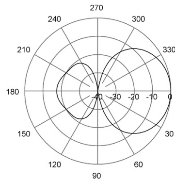
E-Plane | 160 MHz
